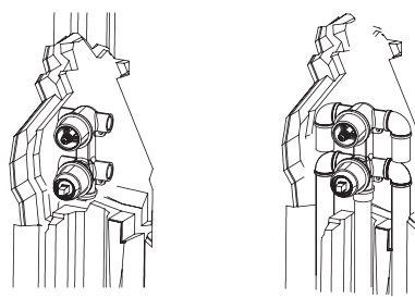
Подключение смесителя на 3 выхода
